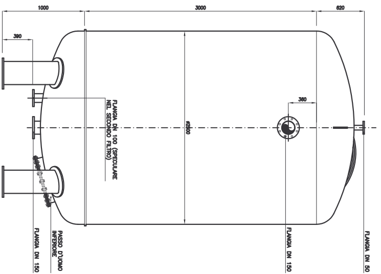
VISTA B
