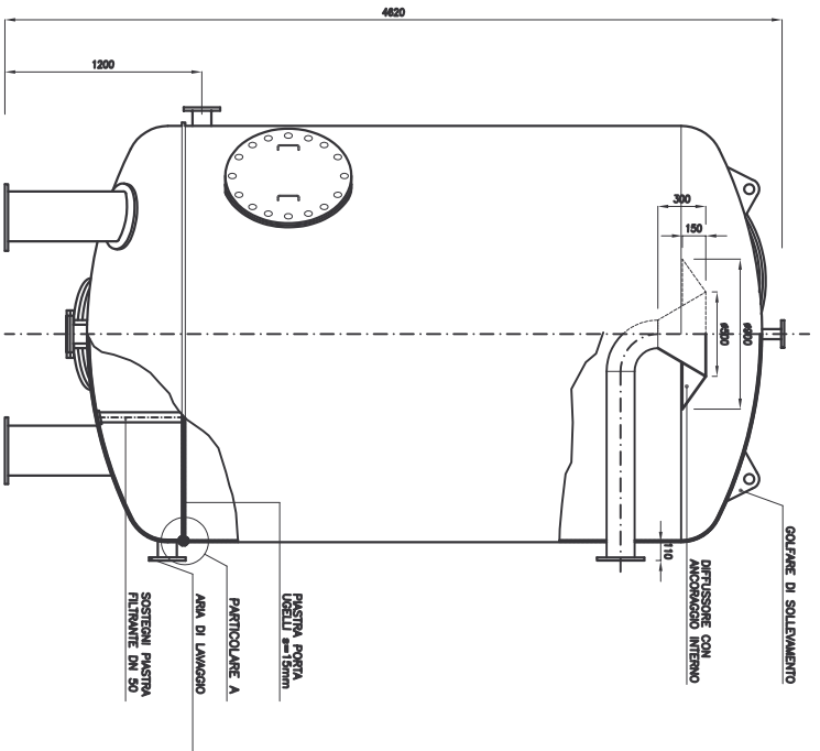
VISTA A
