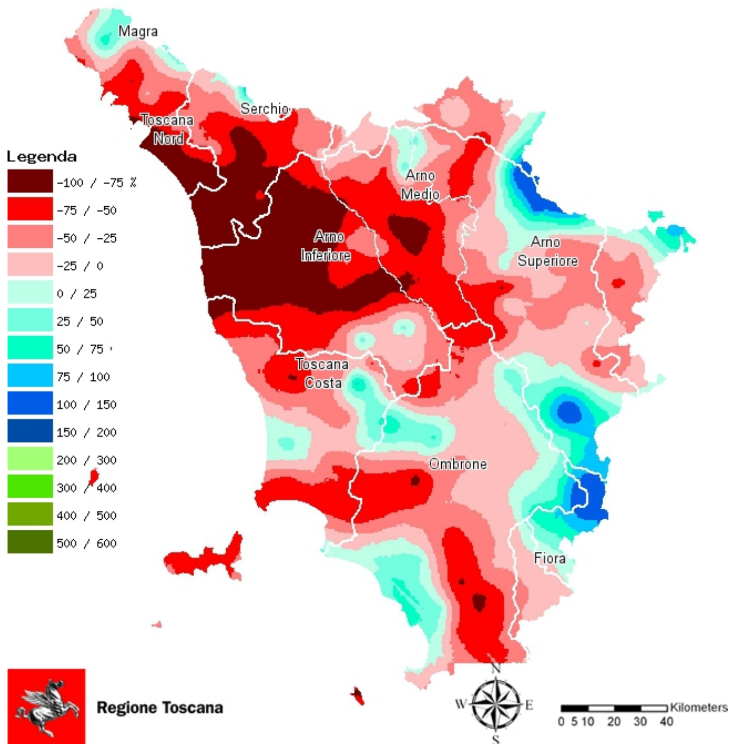
Fig. 2 - Confronto tra le precipitazioni (%) di luglio 2016 con le medie di luglio del periodo 1986-2015
