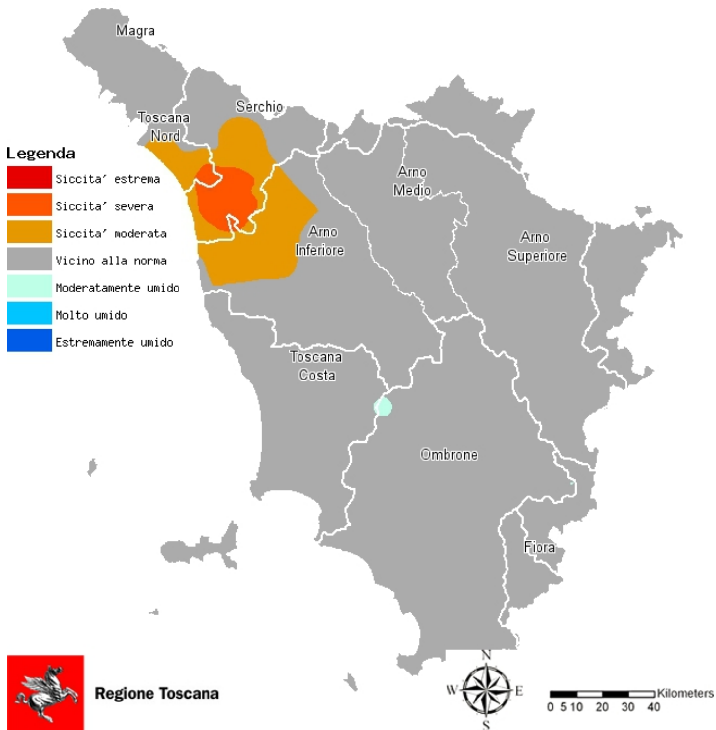
Fig. 6 - Distribuzione dell'indice SPI (Standardized Precipitation Index) al mese di luglio 2016
