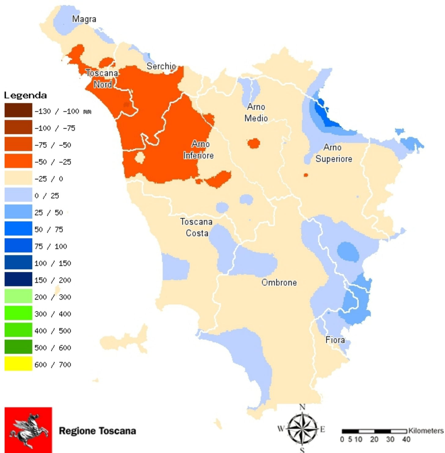
Fig. 3 - Confronto tra le precipitazioni (mm) di luglio 2016 con le medie di luglio nel periodo 1986-2015
