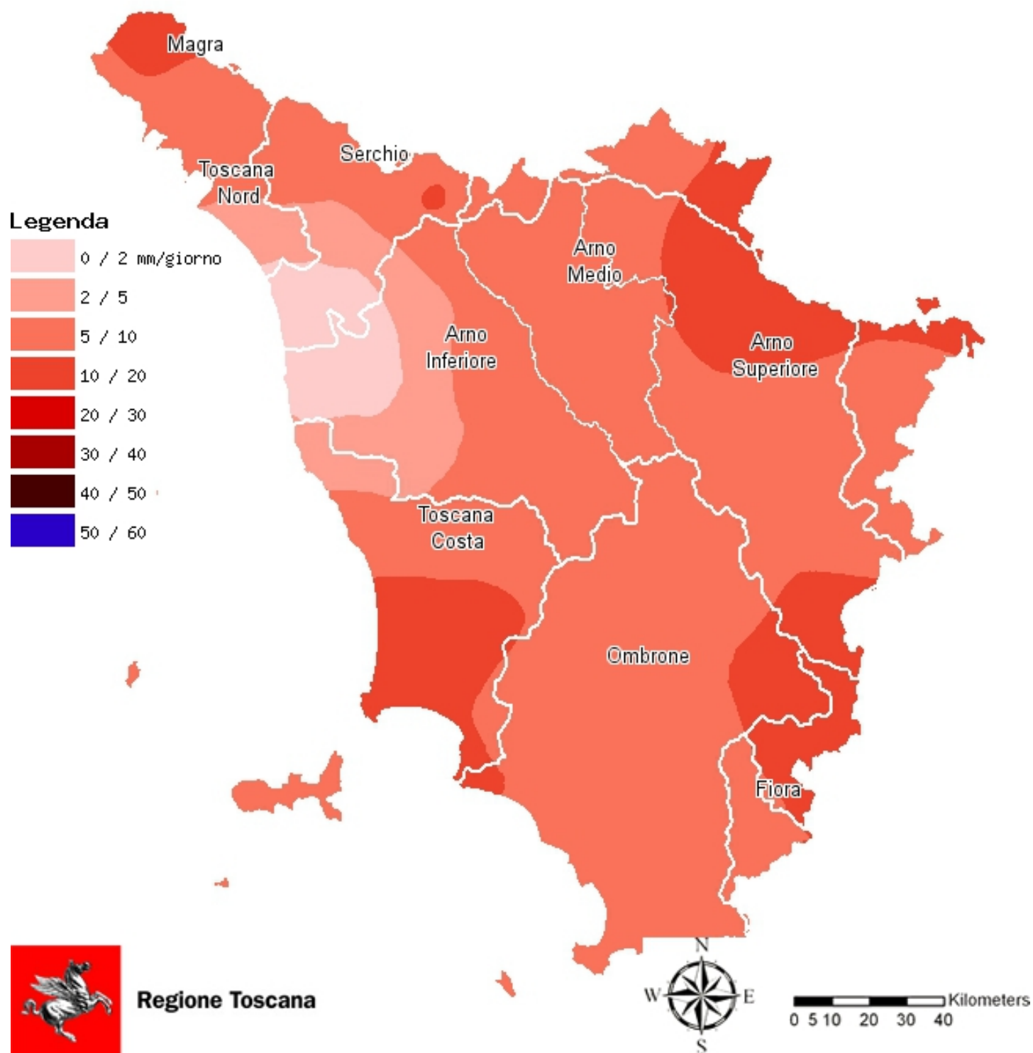
Fig. 5 - Distribuzione dell'intensità media di pioggia (mm/gg piovosi) del mese di luglio 2016
