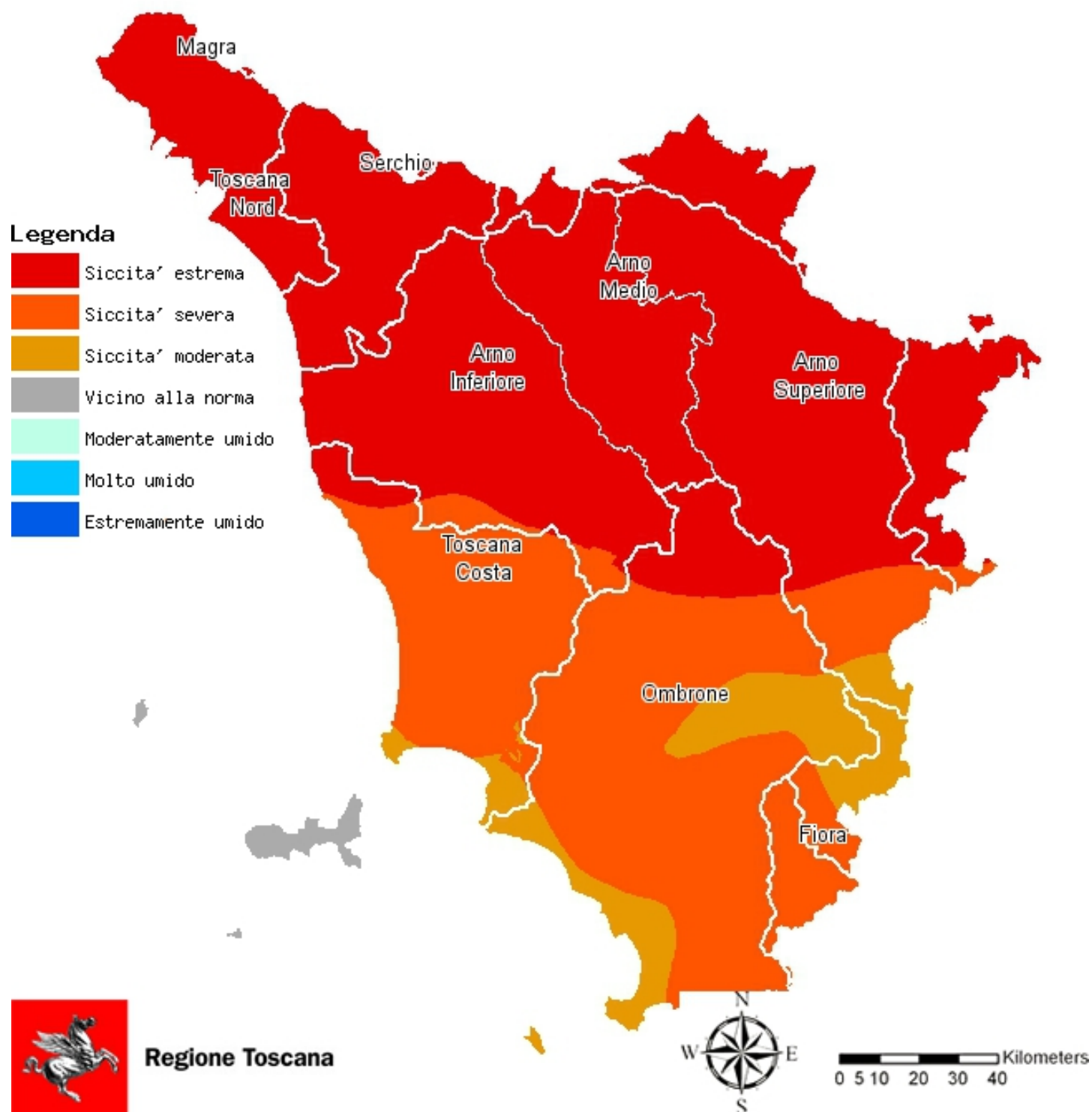
Fig. 6 - Distribuzione dell'indice SPI (Standardized Precipitation Index) al mese di dicembre 2016
