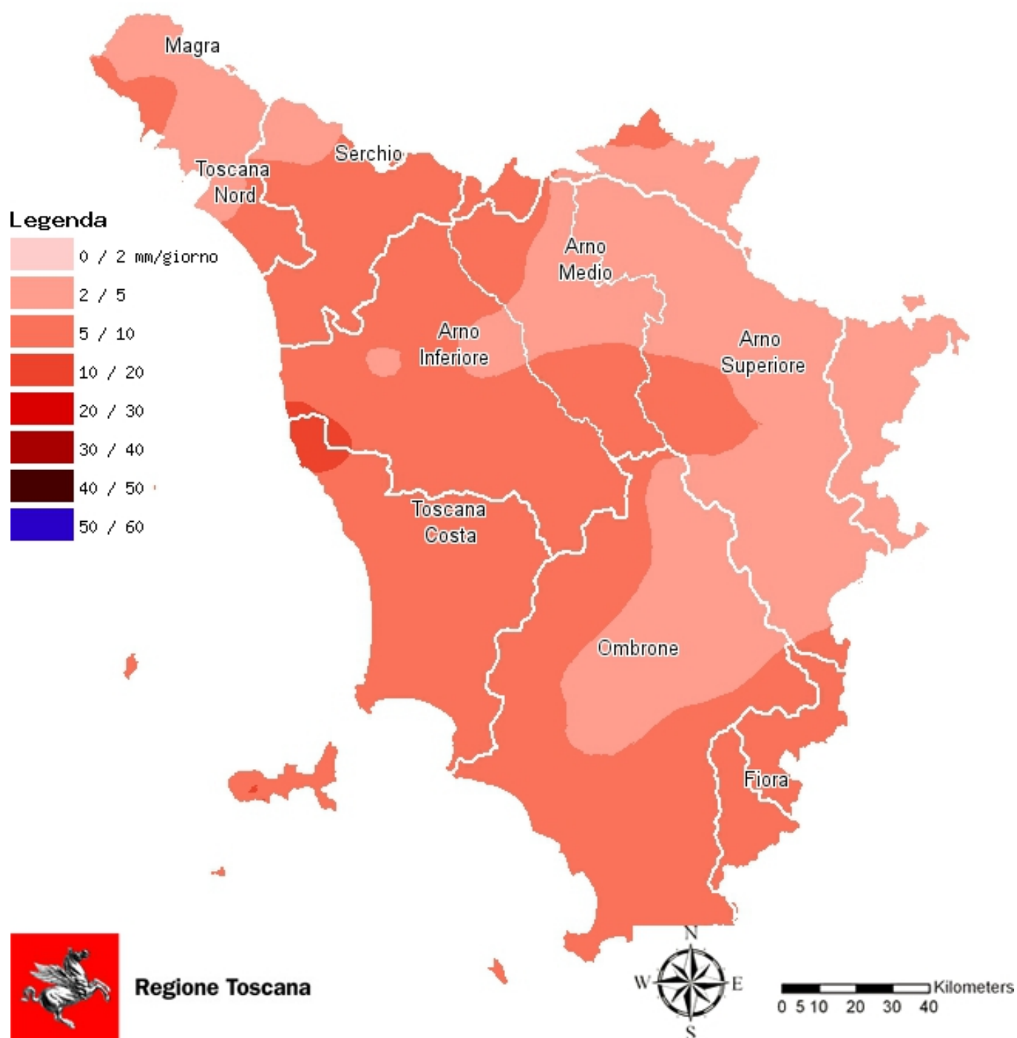
Fig. 5 - Distribuzione dell'intensità media di pioggia (mm/gg piovosi) del mese di dicembre 2016
