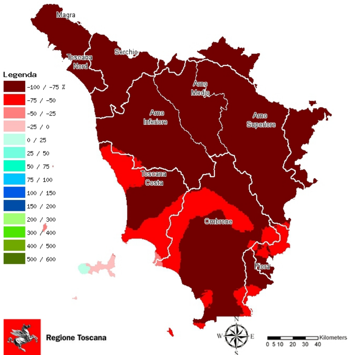
Fig. 2 - Confronto tra le precipitazioni (%) di dicembre 2016 con le medie di dicembre del periodo 1986-2015
