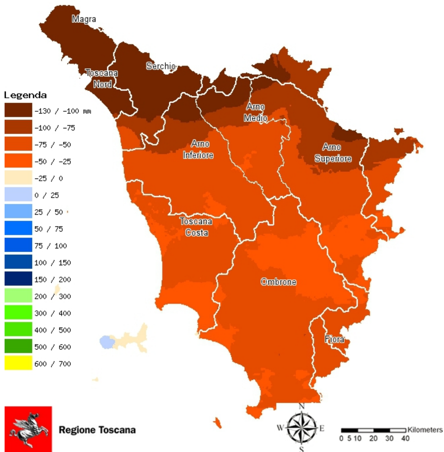
Fig. 3 - Confronto tra le precipitazioni (mm) di dicembre 2016 con le medie di dicembre nel periodo 1986-2015
