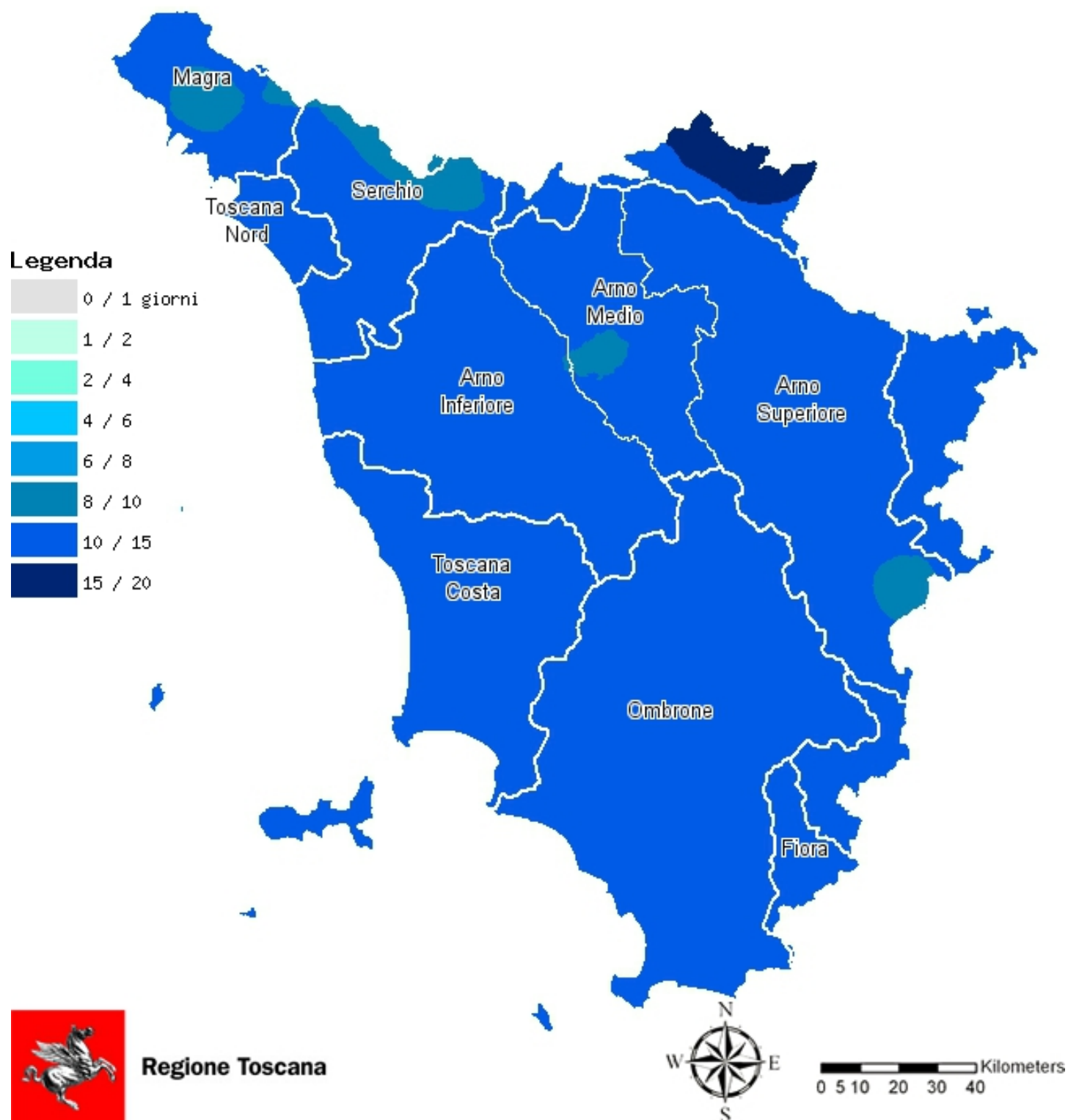
Fig. 4 - Distribuzione dei giorni piovosi ( \geq 1\text{mm} ) del mese di febbraio 2018
