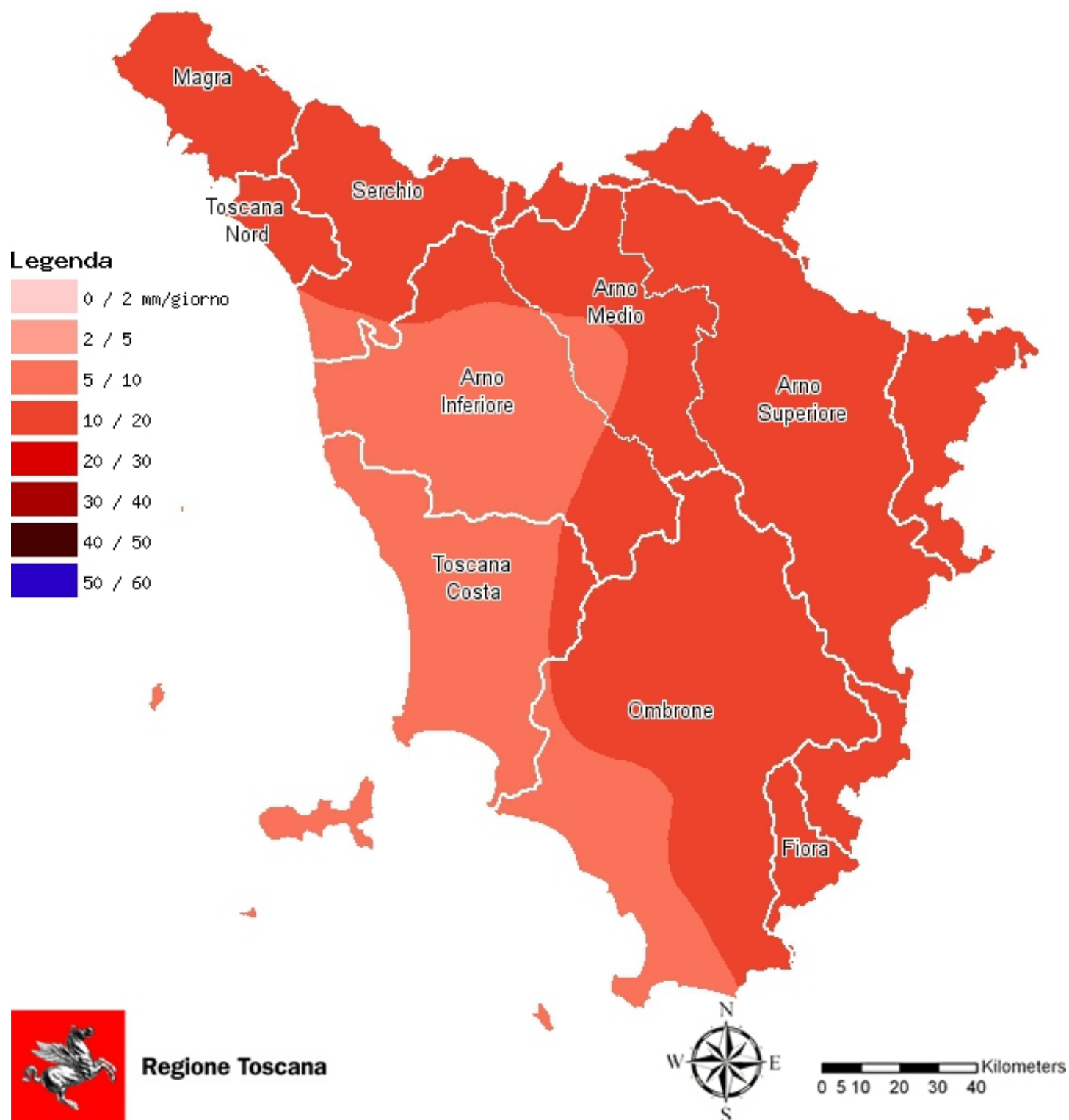
Fig. 5 - Distribuzione dell'intensità media di pioggia (mm/gg piovosi) del mese di febbraio 2018
