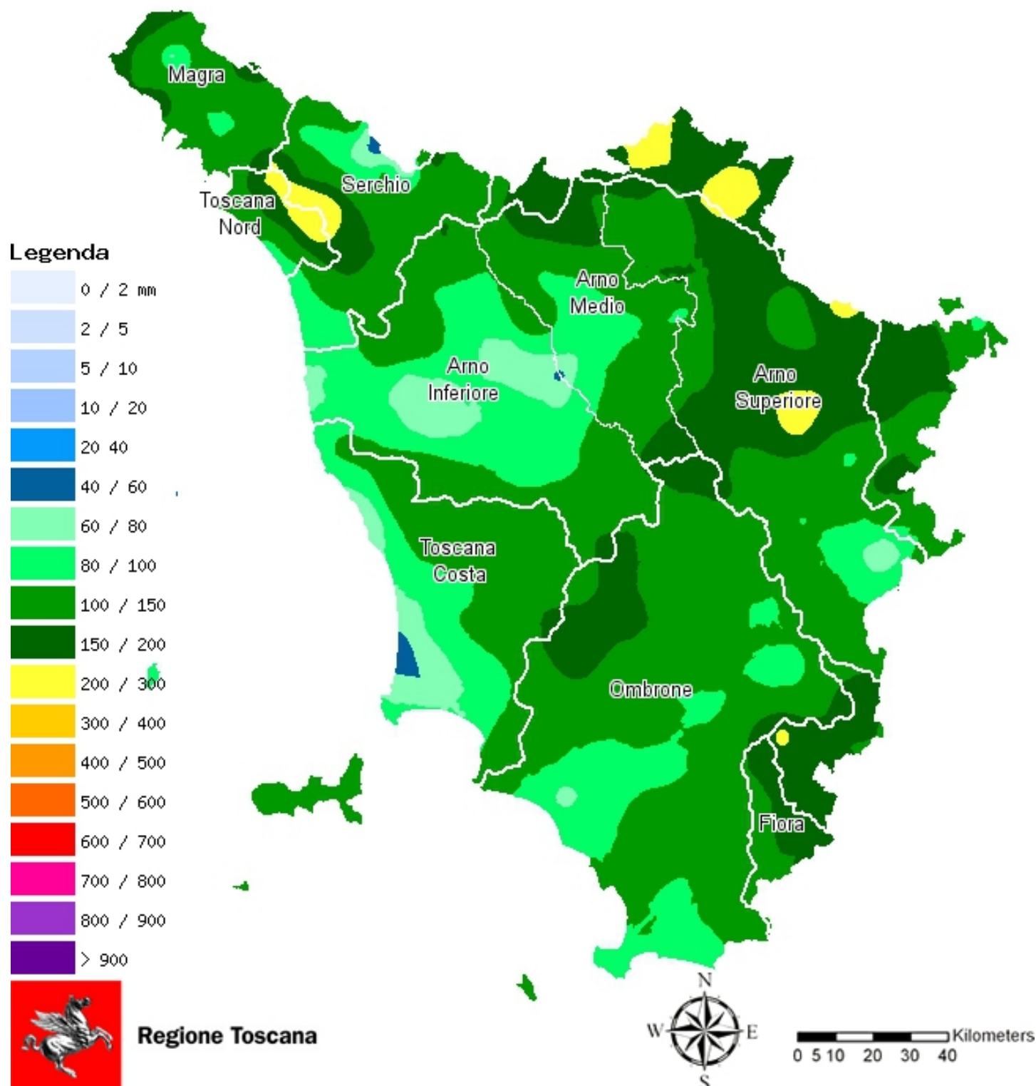
Fig. 1 - Distribuzione delle piogge del mese di febbraio 2018
