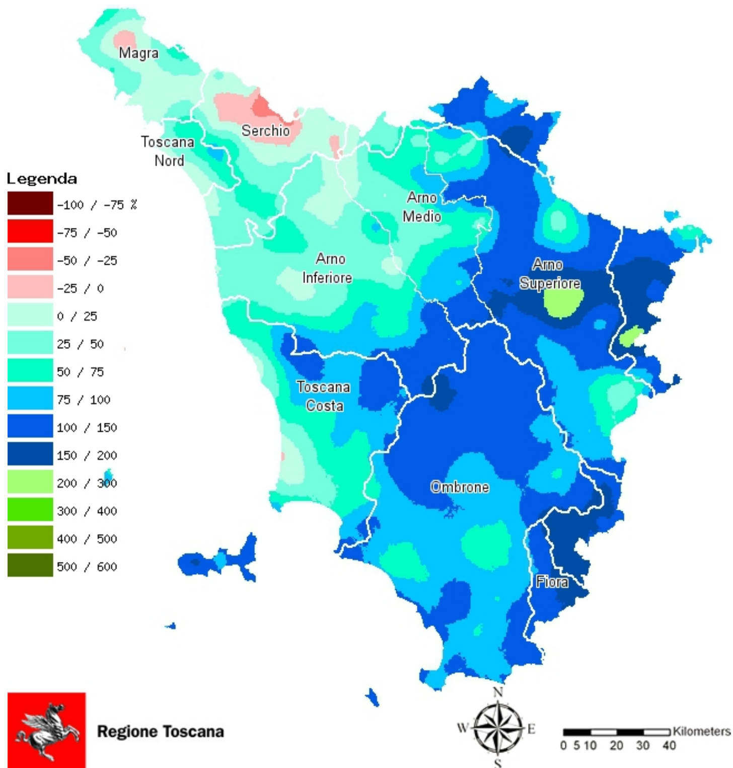
Fig. 2 - Confronto tra le precipitazioni (%) di febbraio 2018 con le medie di febbraio del periodo 1988-2017
