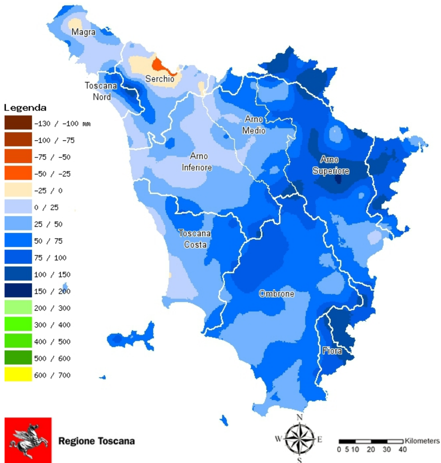
Fig. 3 - Confronto tra le precipitazioni (mm) di febbraio 2018 con le medie di febbraio nel periodo 1988-2017
