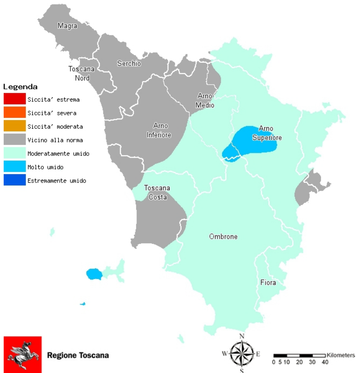
Fig. 6 - Distribuzione dell'indice SPI (Standardized Precipitation Index) al mese di febbraio 2018
