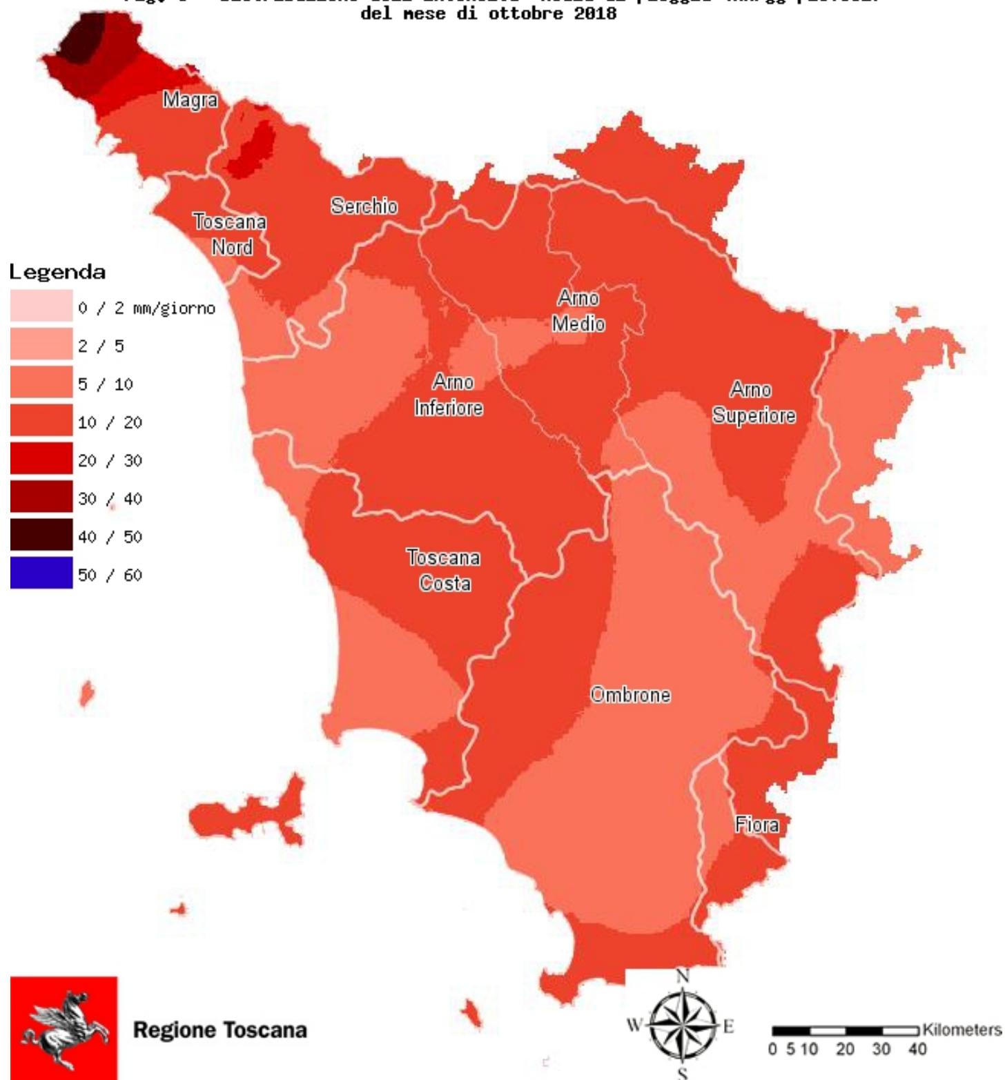
Fig. 5 - Distribuzione dell'intensità media di pioggia (mm/gg piovosi) del mese di ottobre 2018
