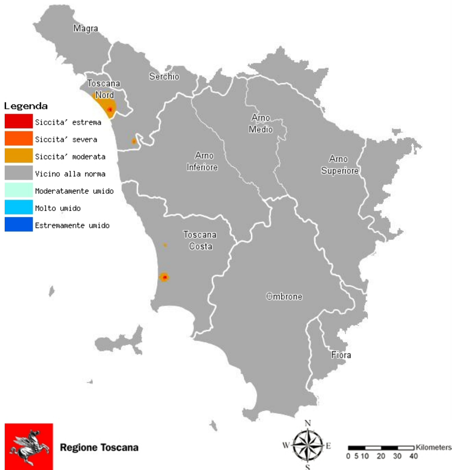
Fig. 6 - Distribuzione dell'indice SPI (Standardized Precipitation Index) al mese di ottobre 2018
