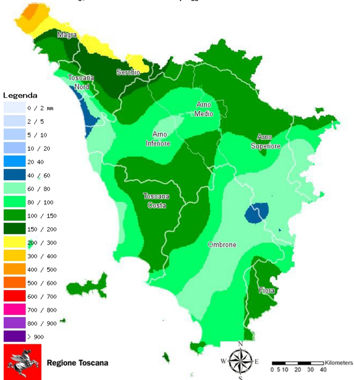
Fig. 1 - Distribuzione delle piogge del mese di ottobre 2018
