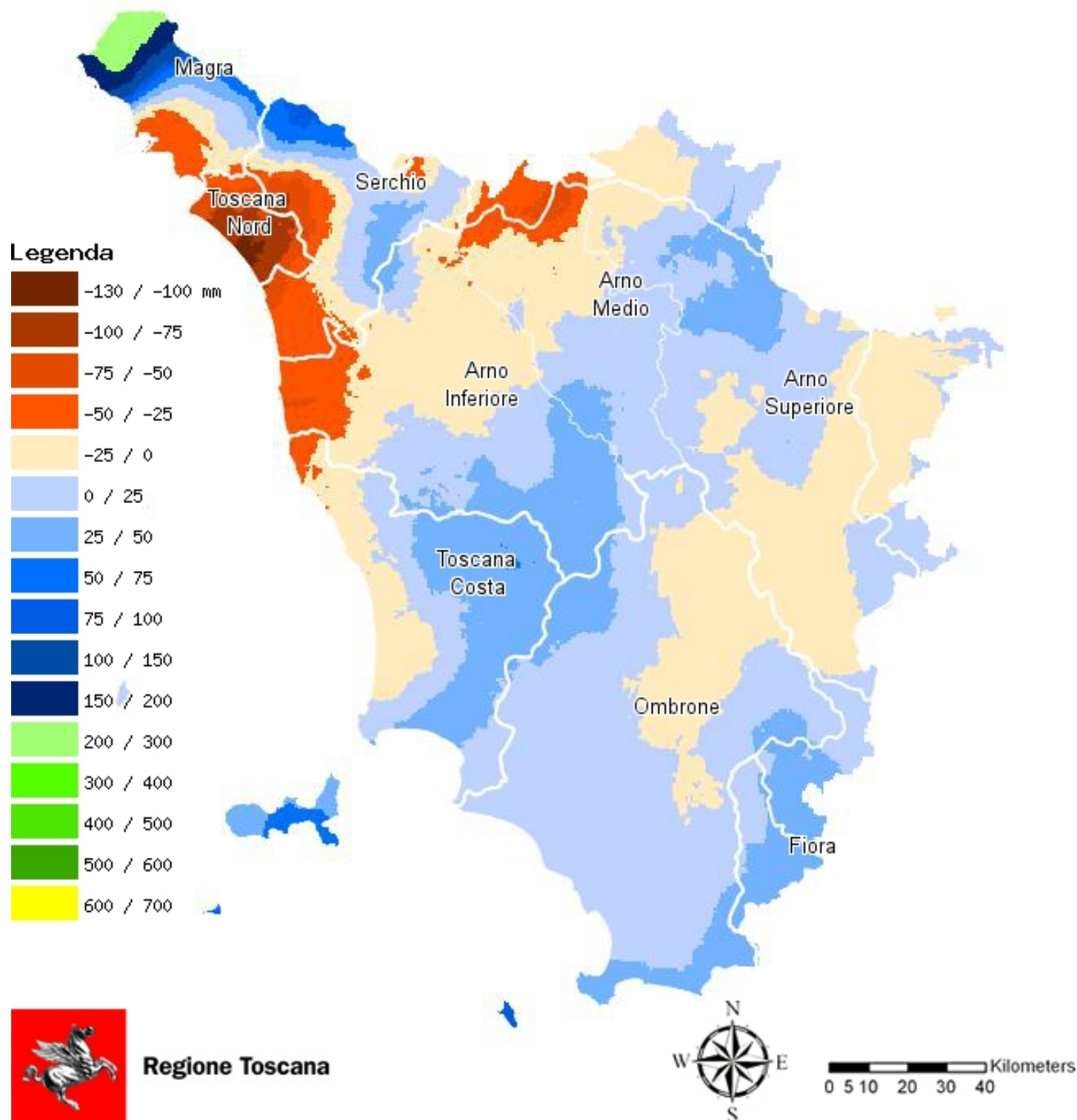
Fig. 3 - Confronto tra le precipitazioni (mm) di ottobre 2018 con le medie di ottobre nel periodo 1988-2017
