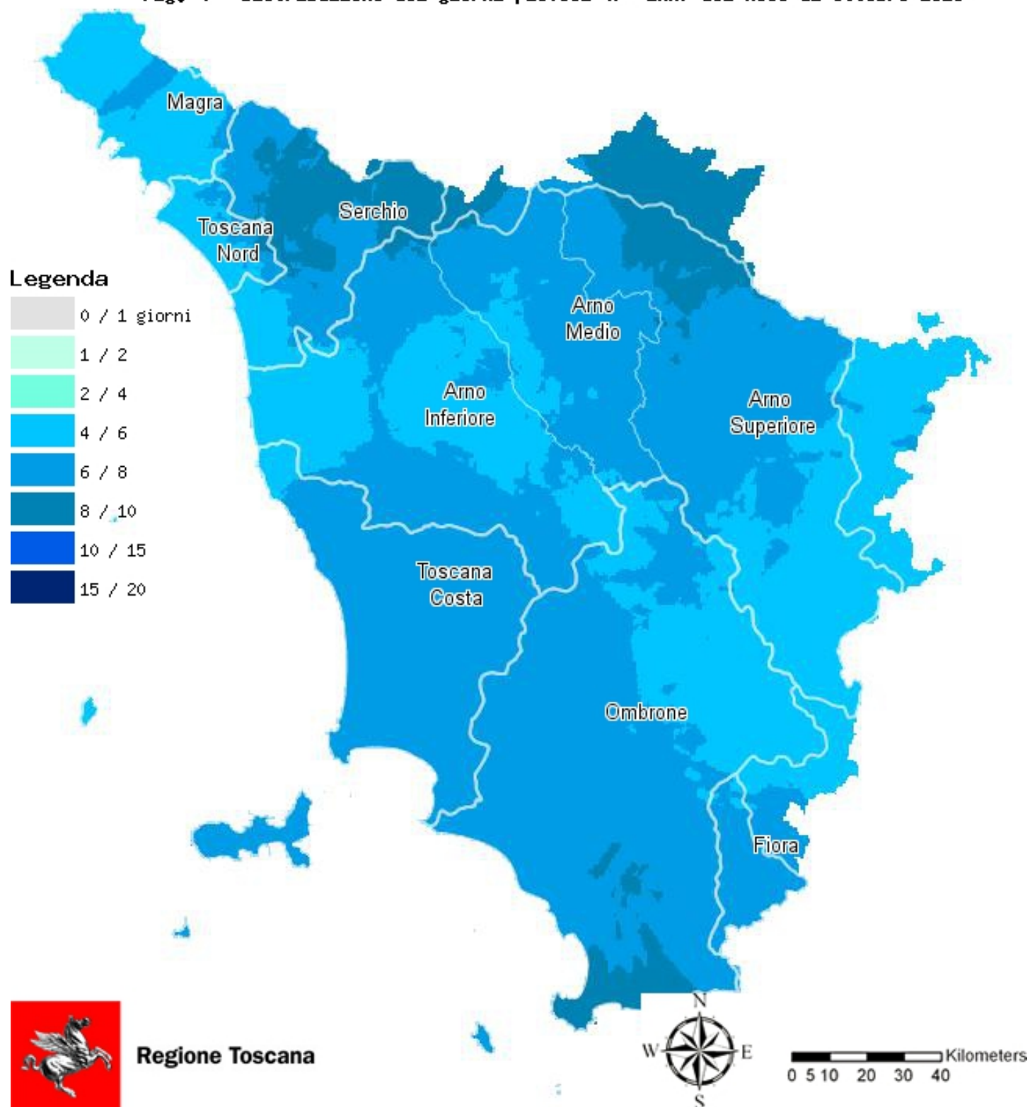
Fig. 4 - Distribuzione dei giorni piovosi ( \geq 1\text{mm} ) del mese di ottobre 2018
