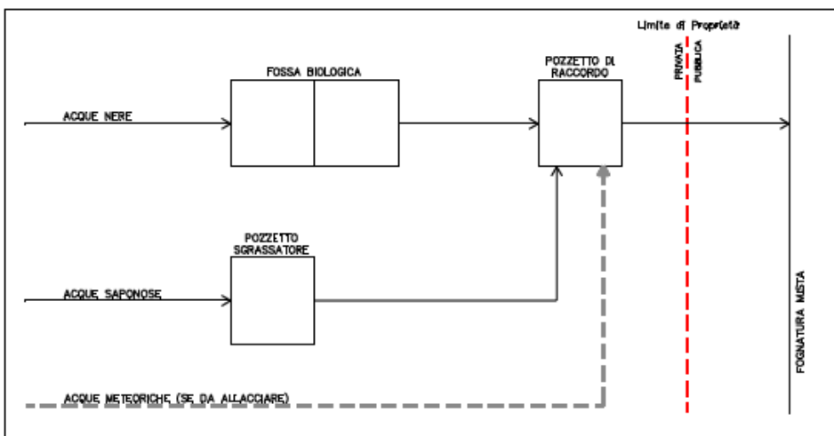
SCHEMA TIPO DI ALLACCIAMENTO DI SCARICHI ACQUE REFLUE DOMESTICHE A FOGNATURA MISTA
