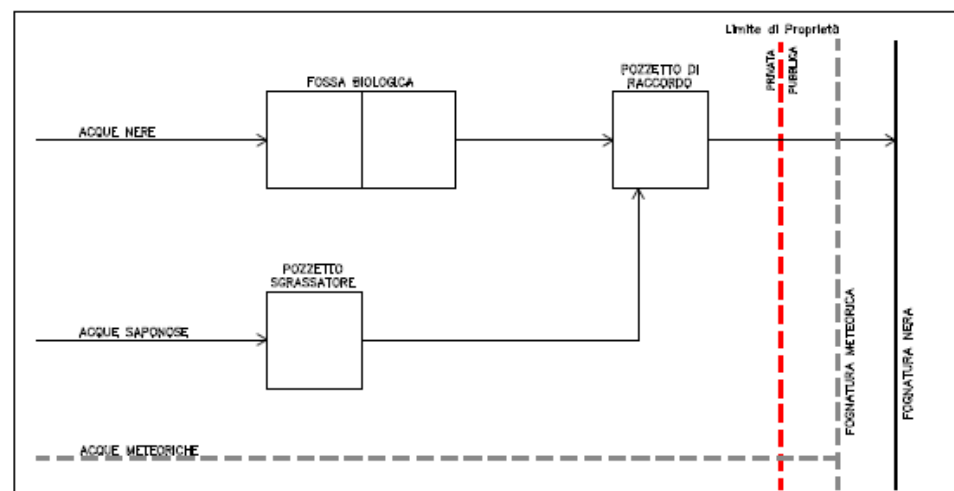
SCHEMA TIPO DI ALLACCIAMENTO DI SCARICHI ACQUE REFLUE DOMESTICHE A FOGNATURA NERA
